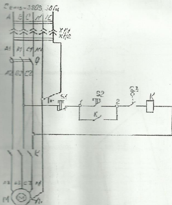
Рисунок 5 – Схема электрическая принципиальная машины СО-313
