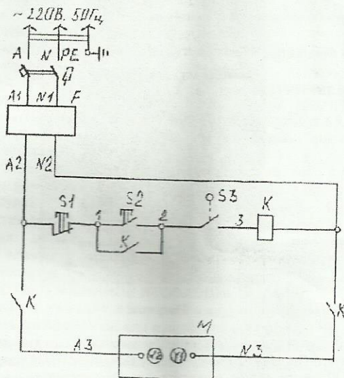
Рисунок 6 –Схема электрическая принципиальная машины СО-313.1
