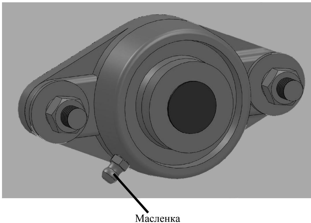
Рисунок 12 – Техническое обслуживание корпусных подшипниковых узлов
