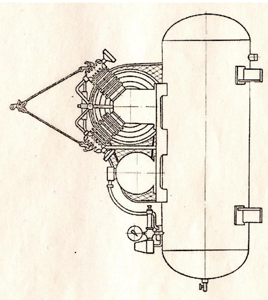
Рис. 20. Схема строповки компрессора модель С416М.
