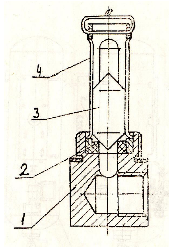
Рис. 11. Влаоудалитель: 1 – корпус; 2 – седло; 3 – клапан; 4 – направляющая.
