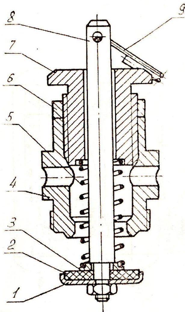
Рис. 9. Пневморазгрузитель.
