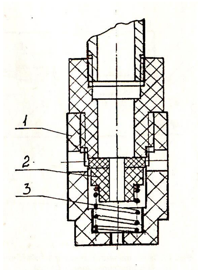
Рис. 14. Обратный клапан. 1 – корпус; 2 – клапан; 3 – пружина.
