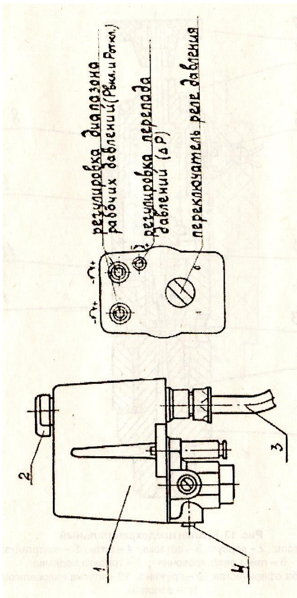
Рис. 12. Реле давления. 1 – кожух; 2 – переключатель; 3 – кабель; 4 – заглушка
