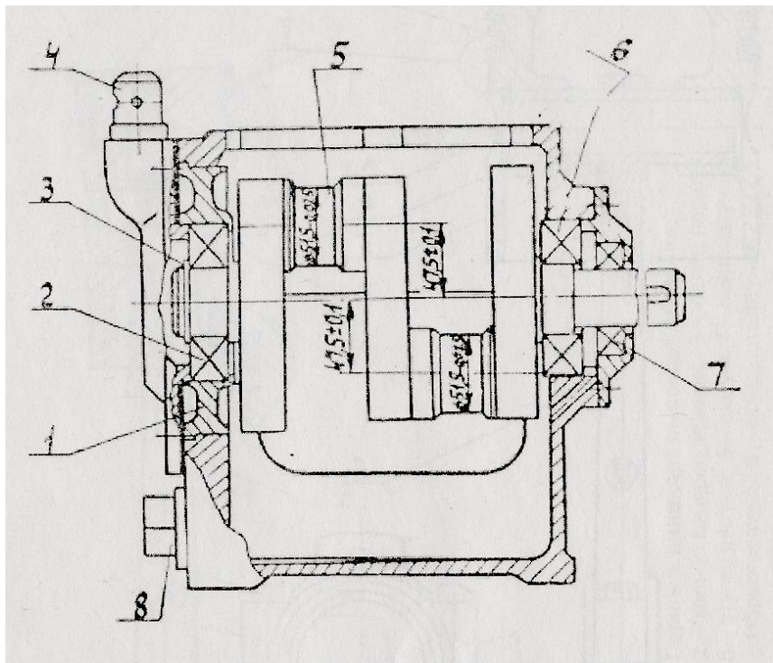
Рис. 5. Картер:
