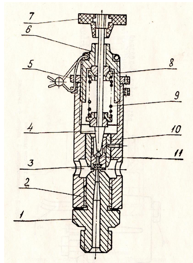
Рис. 13. Клапан предохранительный.
